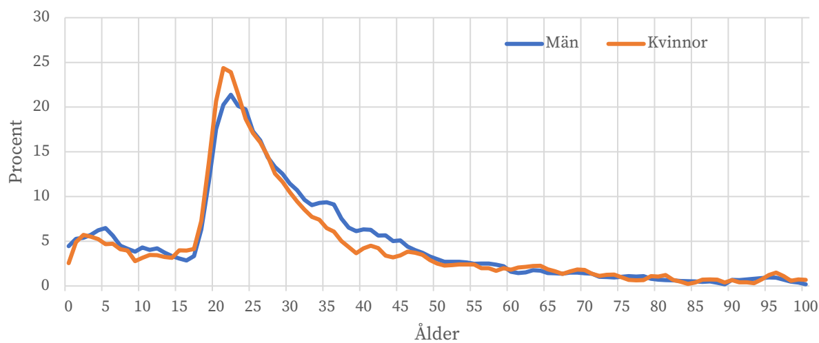
Figur 12. Utflyttningsrisk 2020–2022
